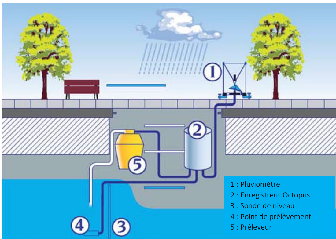
Intégration du pluviomètre à une chaîne de mesure
